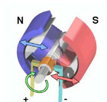
Мал. 1. Принцип роботи двигуна постійного струму
