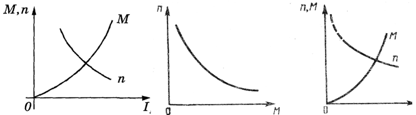
Мал. 6. Характеристики двигуна з послідовним збудженням: а – швидкісна; б – механічна; в - робочі
